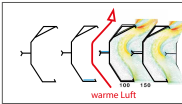
Ursprüngliche Geometrie Version 2 Cv= 0,414 des freien Querschnitts
