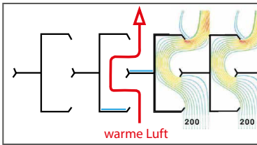
Ursprüngliche Geometrie Version 1 Cv= 0,296 des freien Querschnitts
